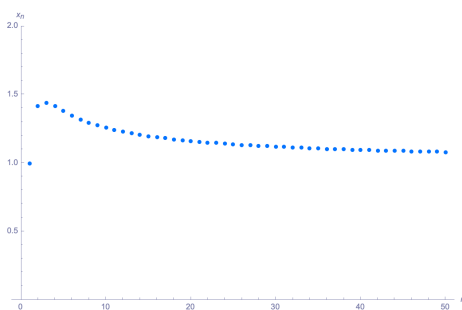
Fig. 3.3: x_n = \sqrt[n]{n}
