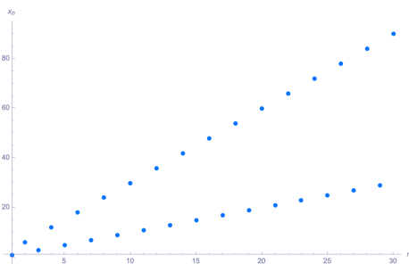
Fig. 3.7: x_n = [2 + (-1)^n]n
